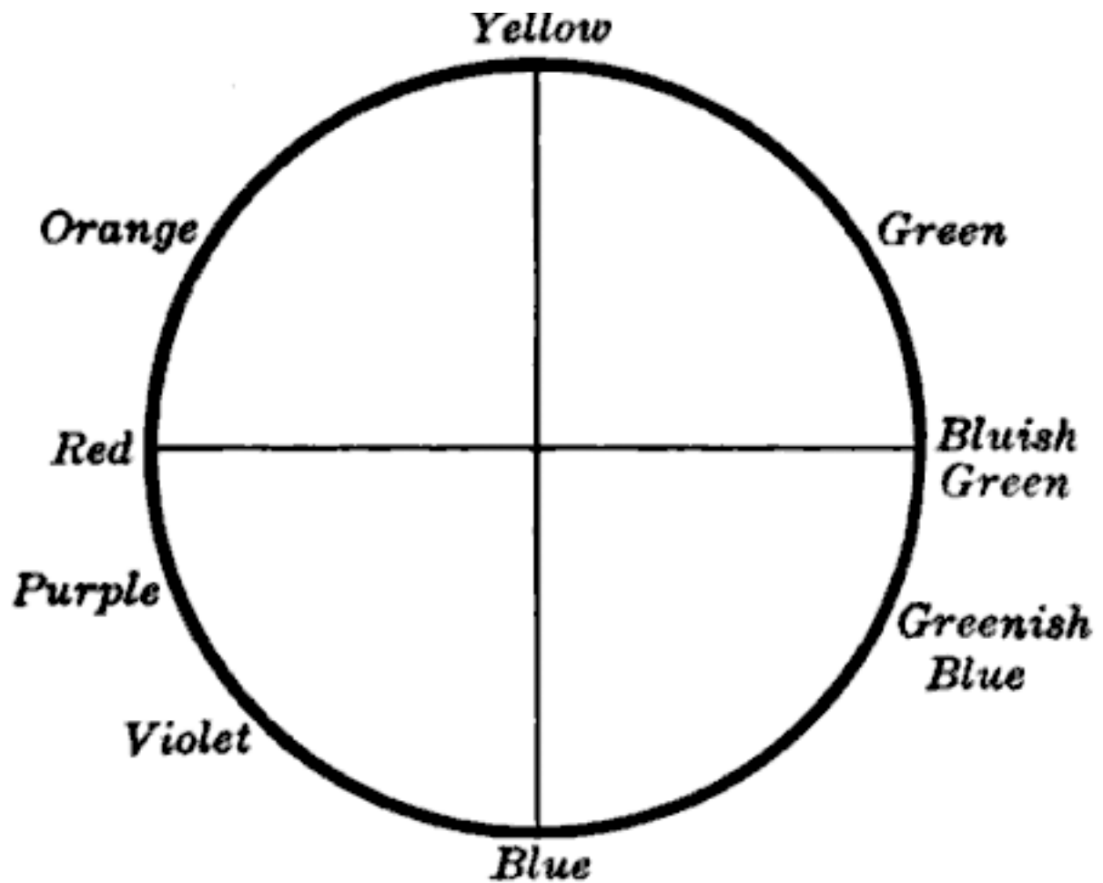
FIG. 23. Color circle
